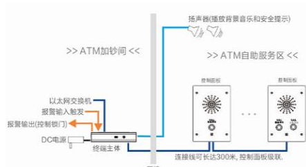
方式一：总线连接
