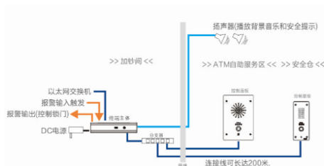
方式二：星型连接
