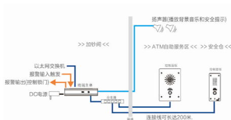
方式二：星型连接
