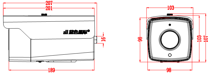
产品尺寸图
